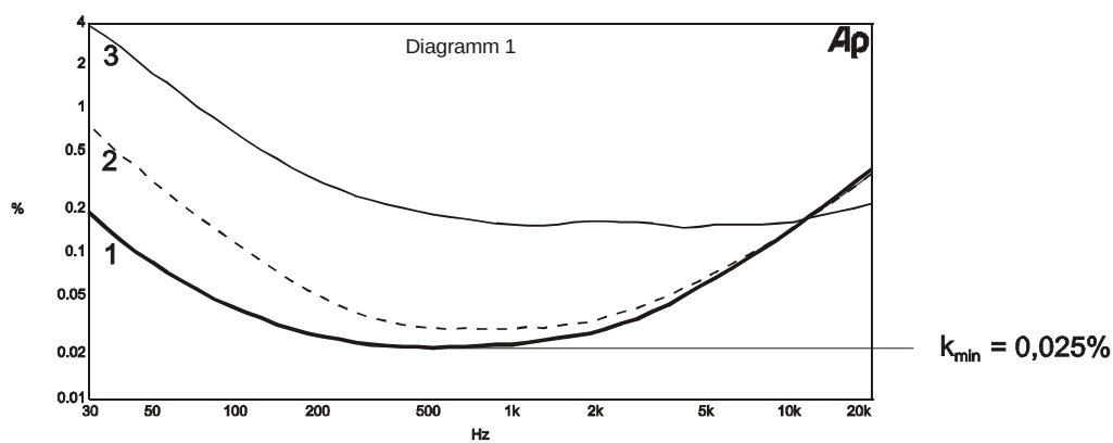
Graph 1: THD at 4V /6Ω from 30Hz~20kHz (いくつかのバイアスセッティング時)
